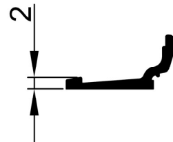
11 - 3202 Cam Çıtası/ Glazig Bead Ağırlık :0,12 kg/m (Weight)
