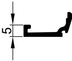
10 - 3133 Cam Çıtası/ Glazig Bead Ağırlık :0,15 kg/m (Weight)
