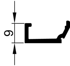
10 - 3244 Cam Çıtası/ Glazig Bead Ağırlık :0,16 kg/m (Weight)
