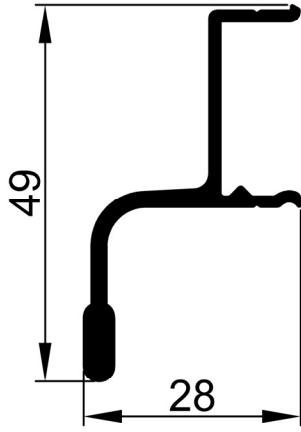
45 SL 51 Damlalık Profili Weatherdrip Profile Ağırlık :0,44 kg/m (Weight)
